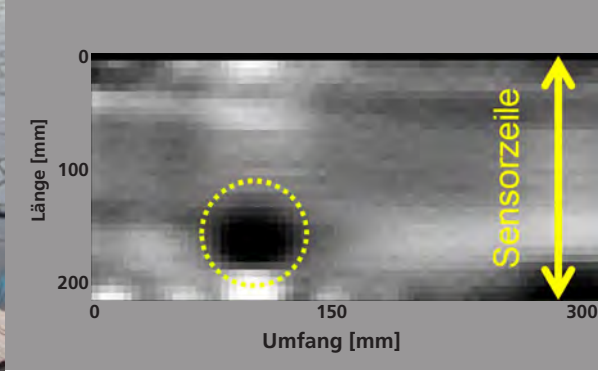
Ergebnisbild eines fehlerhaften Betonmastes
