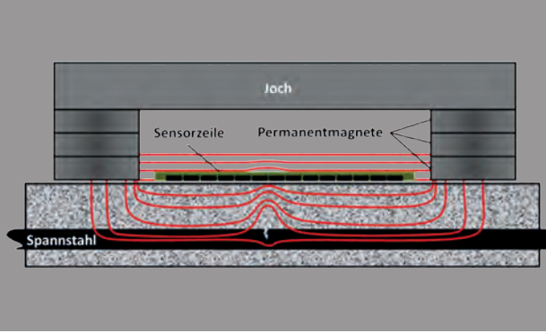
Feldlinienverlauf an beschädigtem Spannstahl
